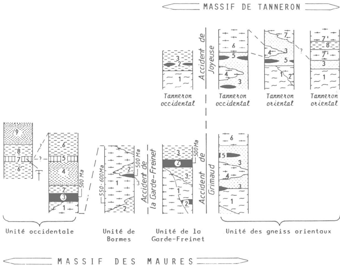
Fig.2 - Essai de lithostratigraphie synthétique des formations métamorphiques de la Provence varisque. Tentative general lithostratigraphy of Variscan Provence metamorphic formations.
