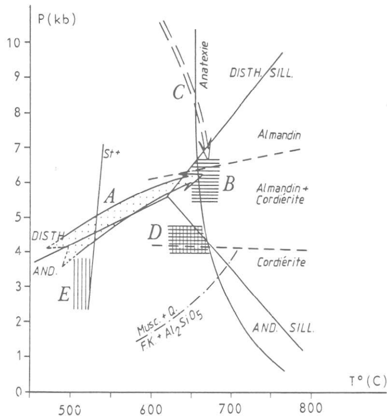
Fig.4 - Diagramme pression-température pour le métamorphisme de la Provence varisque. Temperature-Pressure conditions of Variscan Provence metamorphism.
