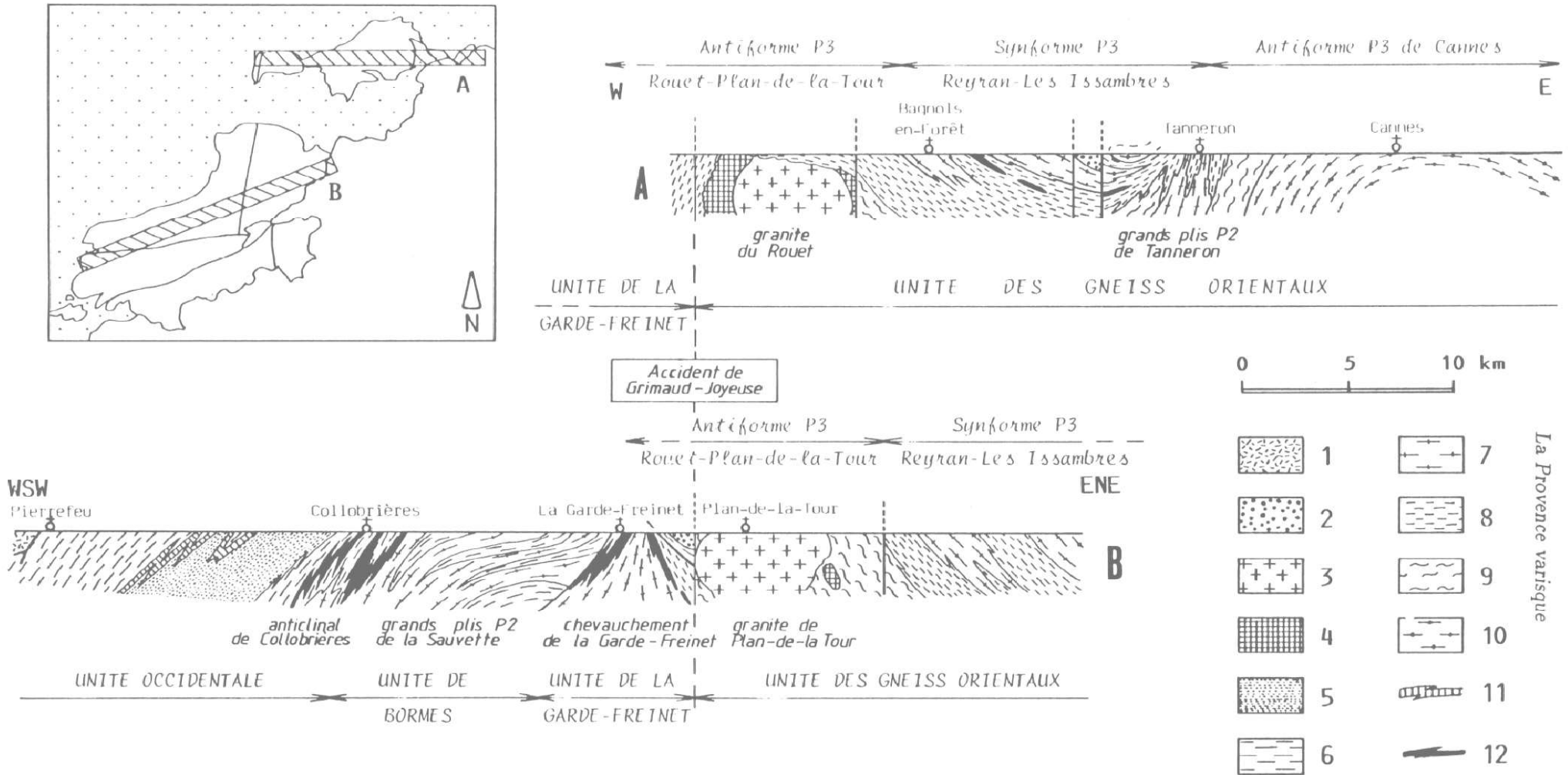
Fig.3 – Coupes géologiques synthétiques. A : Massif de Tanneron ; B : partie nord du Massif des Maures. Synthetic cross-sections. A : Tanneron Massif ; B : Northern Maures Massif
