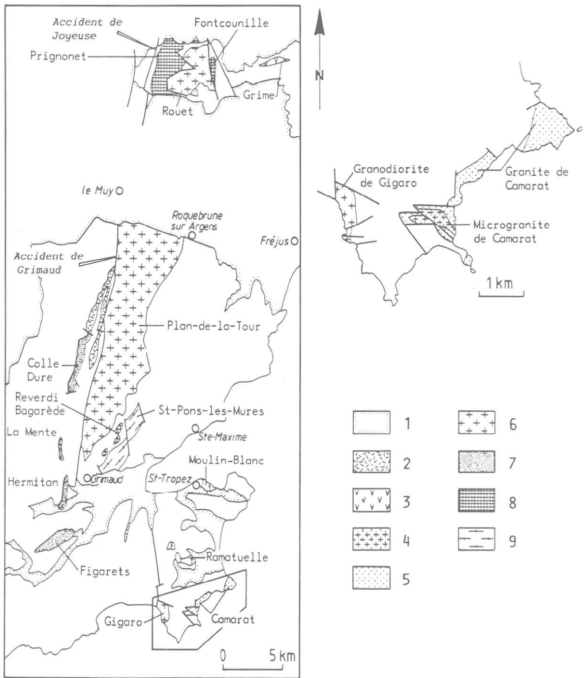
Fig.5 – Les principaux massifs de granitoïdes de la Provence varisque. Main granitoidic massifs of Variscan Provence.
